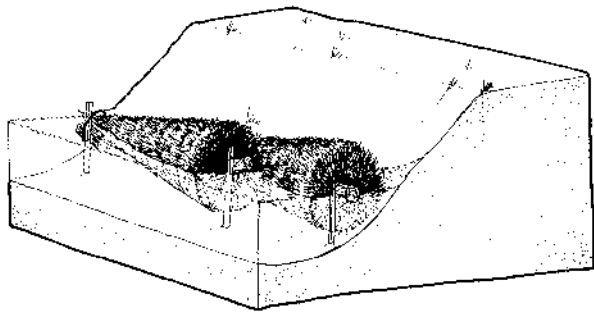
Brush Revetment
